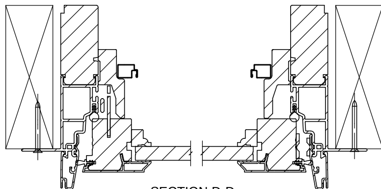
SECTION D-D SCALE 1 : 3
